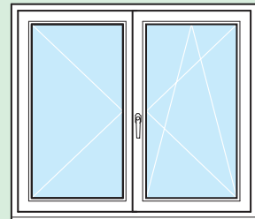
Dreh-Drehkipp-Fenster mit Stulp
