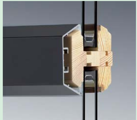
TSP: echte glasteilende Trapezsprosse
