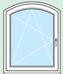
Drehkipp-Fenster Stichbogen
