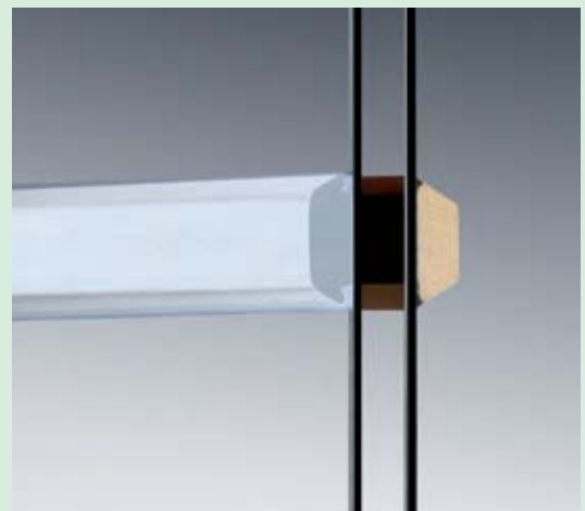
ASP: außen Alu-Sprosse, innen Holz-Trapezsprosse
